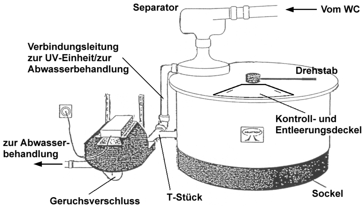
Abbildung 2. Aquatron 4x100 / 4x200, installiert auf einem Sockel
