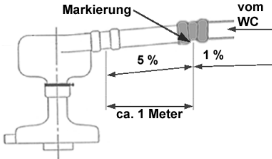
Abbildung 9. Speziell angewinkelte Doppelmuffe für Einlaufrohre über 1 Meter
