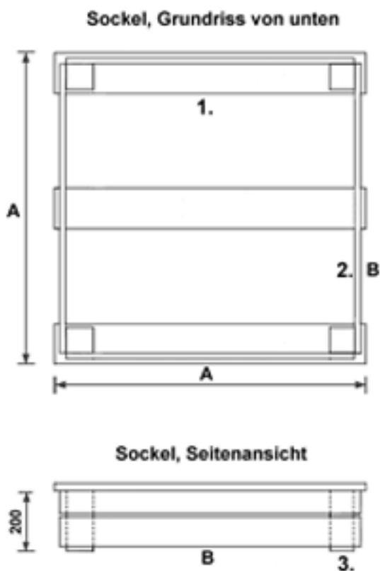
Abbildung 3. Skizze für einen Sockel für das Aquatron 4x100 / 4x200
