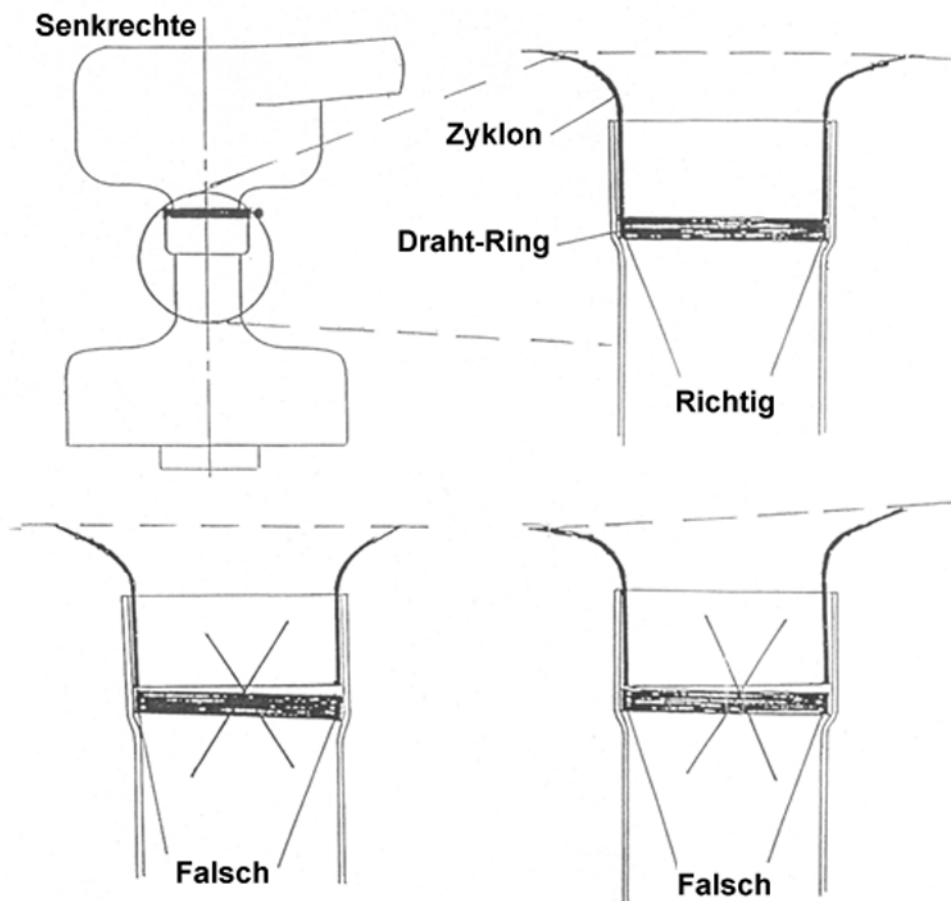
Abbildung 4. Installation des Separators
