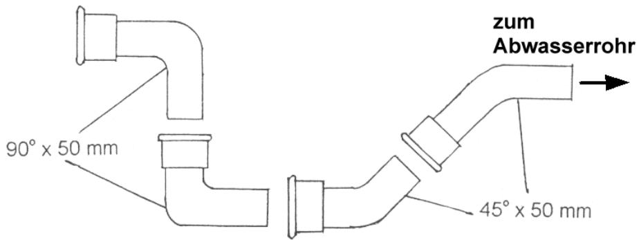
Abbildung 6. Vorschlag für einen Geruchsverschluss
