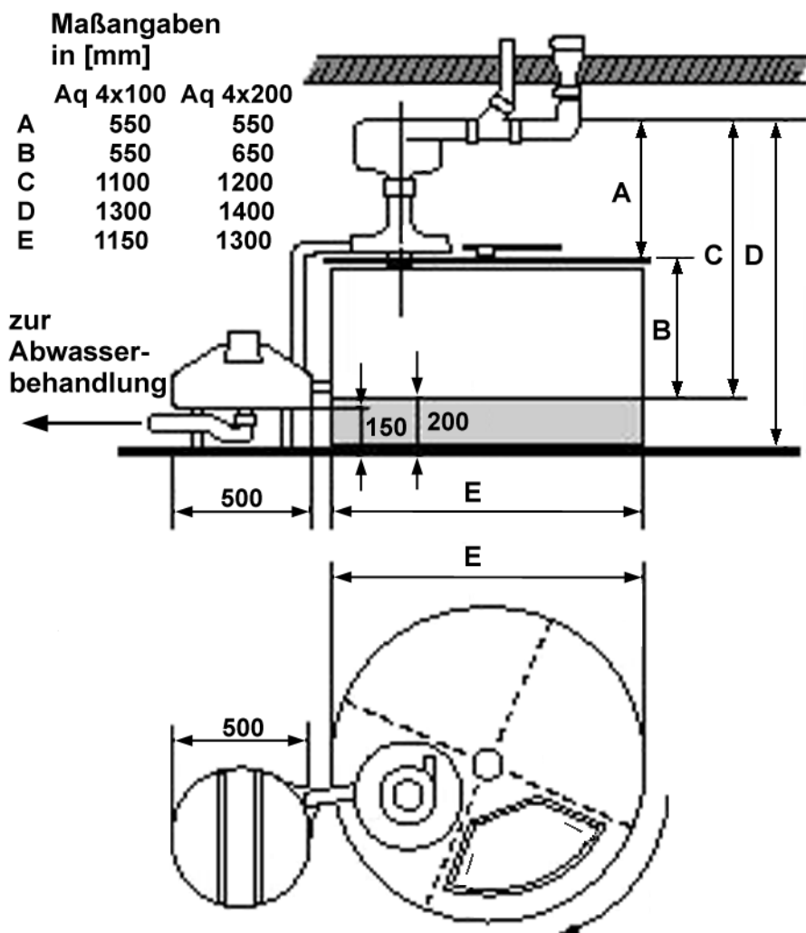
Abbildung 1. Installationsmaße für das Aquatron 4x100 / 4x200
