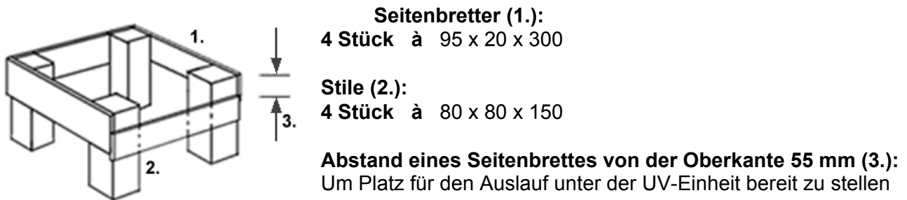
Abbildung 5. Sockel für die UV-Einheit
