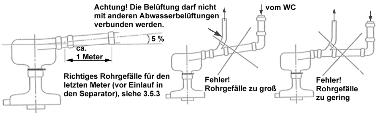
Abbildung 8. Winkeleinstellung am Einlaufrohr vom WC zum Separator
