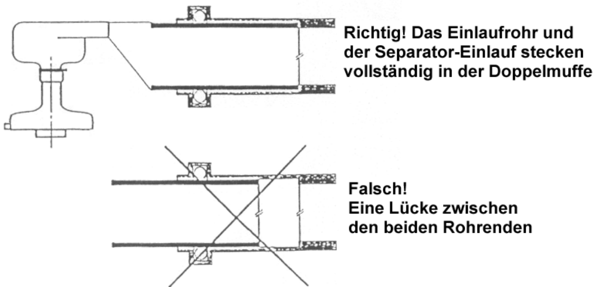
Abbildung 7. Anschluss des Einlaufrohres an den Separator mit einer Doppelmuffe
