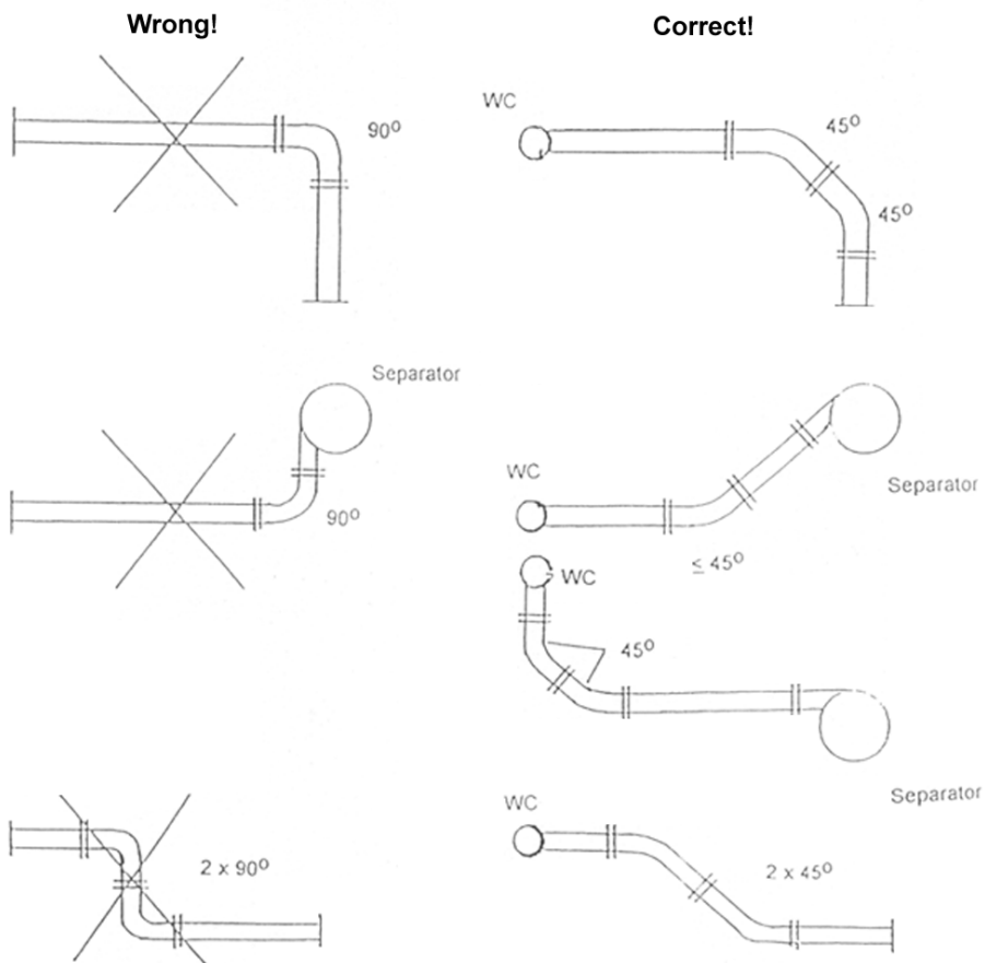
Abbildung 10. Einige Beispiele für horizontale Rohrbögen
