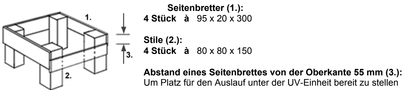
Abbildung 5. Sockel für die UV-Einheit
