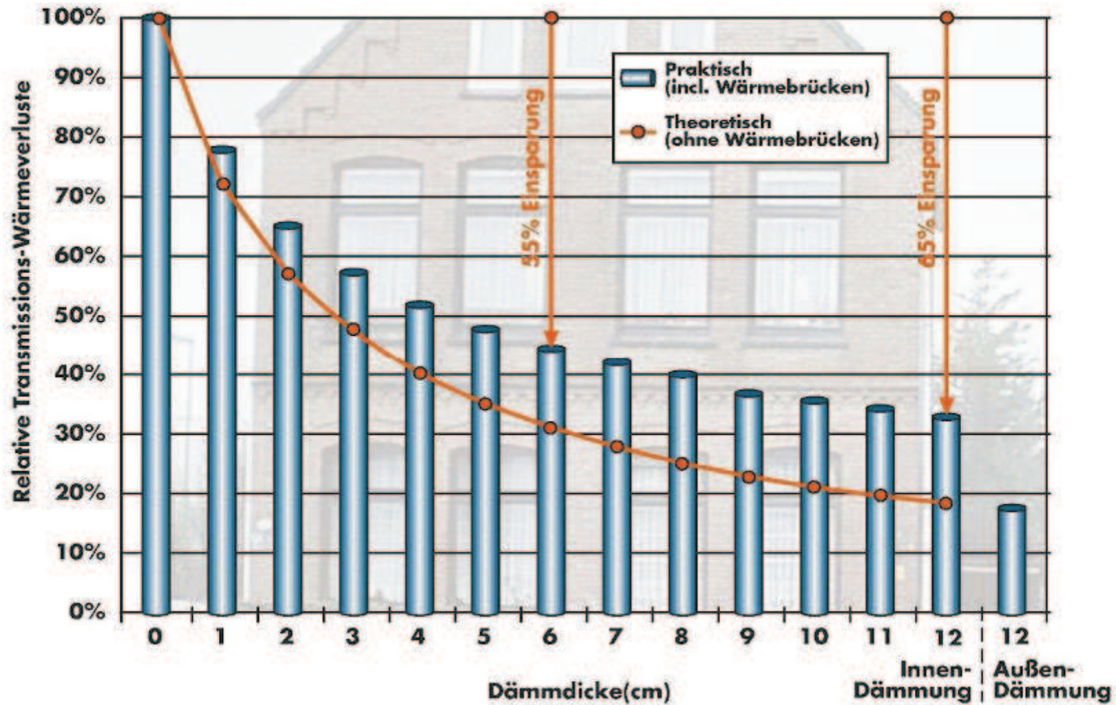
Einsparung durch Innendämmung am Beispiel eines Einfamilienhauses Baujahr 1953
